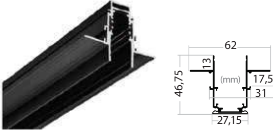
Sıva Altı Alüminyum Ray / Recessed Aluminum Track
